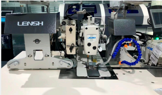
LS7041B 锁式 Lock type
